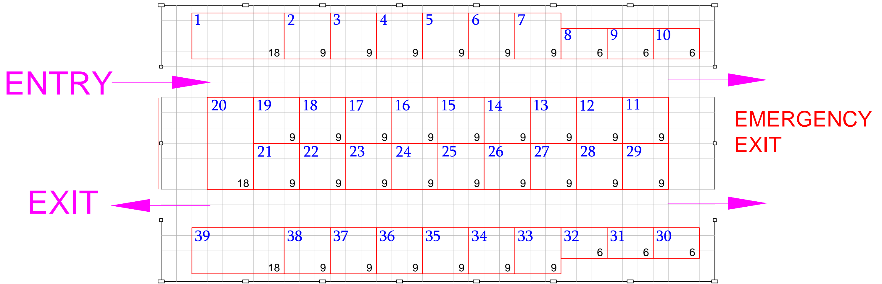
18 x 36m Hangar-M
